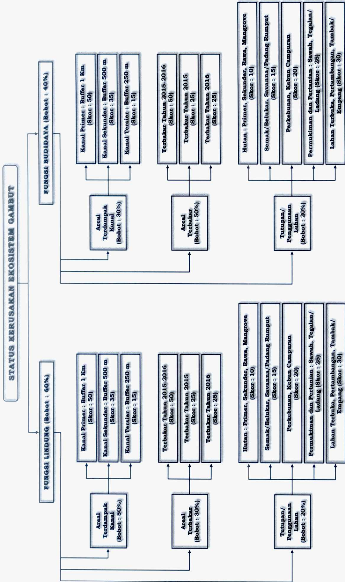
Gambar 2.2 Metodologi Kriteria Penentuan Status Kerusakan Ekosistem Gambut (Metode Skoring dan Pembobotan)
