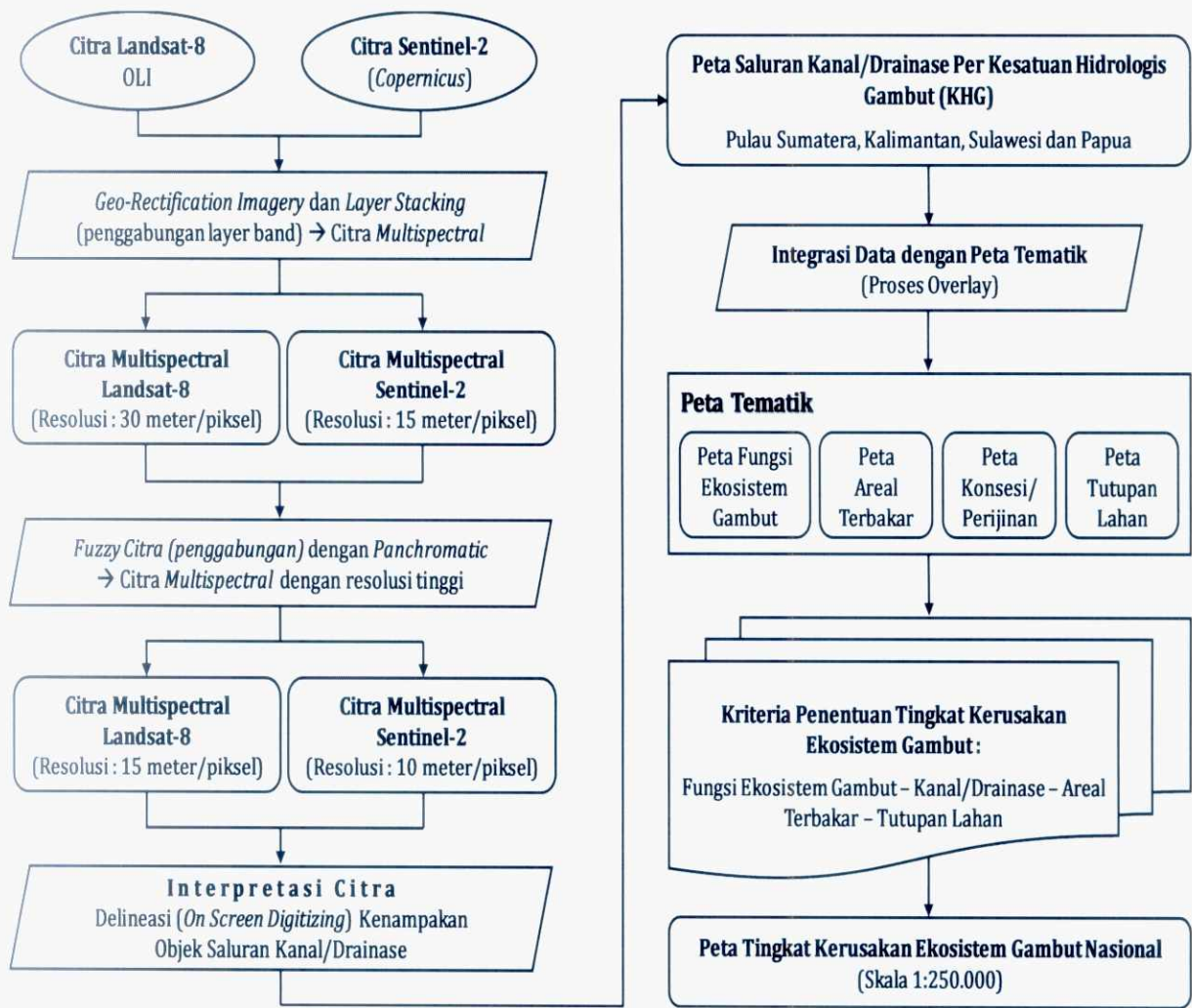
Gambar 2.1. Tahapan Interpretasi dan Analisis Data Spasial Saluran Drainase
